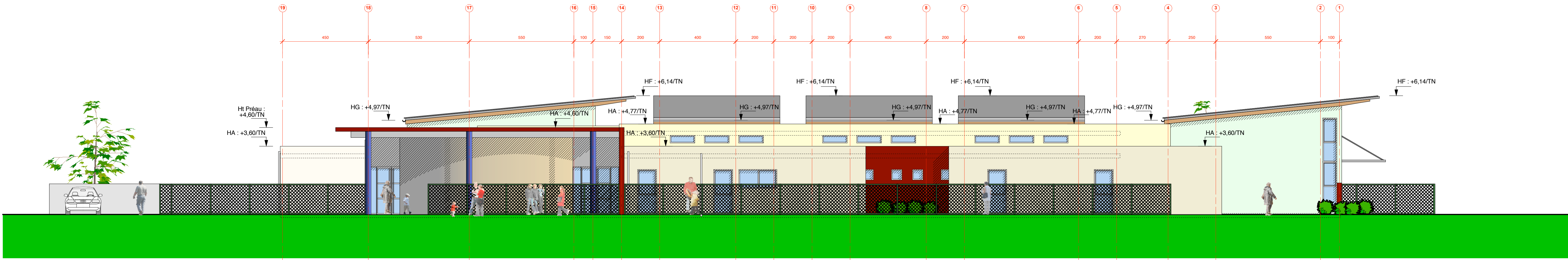
FACADE OUEST SUR RUE
